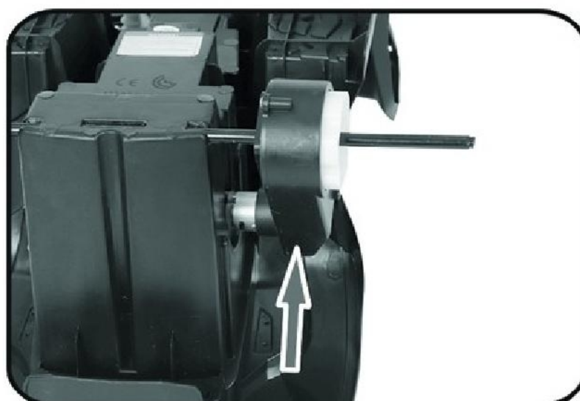
5. Nabacite elektromotor na osovinu
