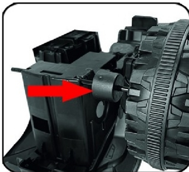
2. Na osovinu ide najpre podloška, točak, plastični odbojnik pa se ista provlači kroz vozilo
