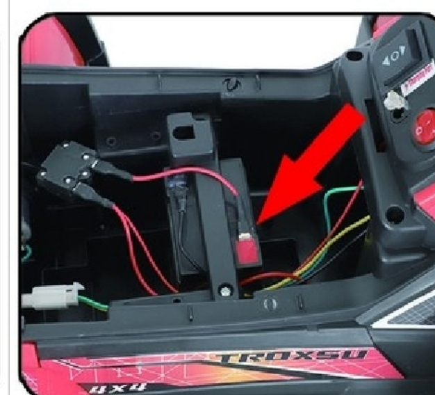
12. Sa crvenog konektora baterije skinite zaštitnu plastiku i povežite slobodnu crvenu žicu
