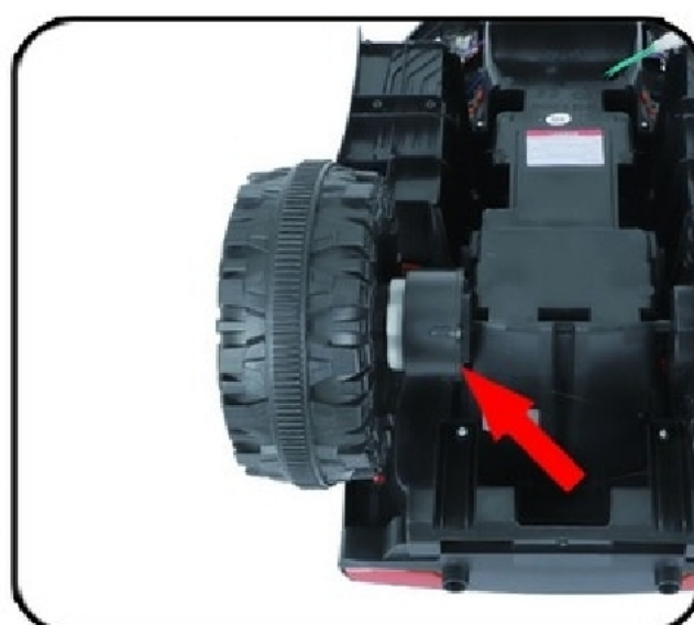
3. Sa druge strane osovinu provucite kroz elektromotor pa nabacite drugi točak
